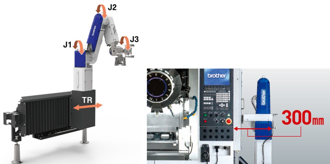
Brother 省人化自動上下料夾持装置 BV-7
