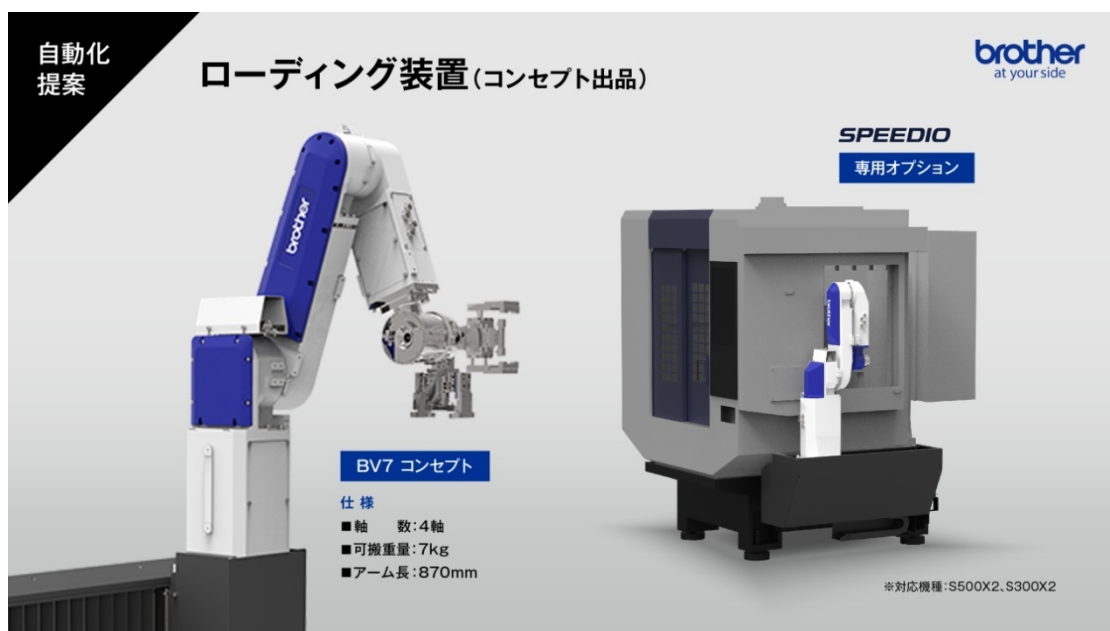
Brother 省人化自動上下料夾持装置 BV-7
